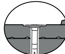
Frapper le clou-vis avec la rondelle jusqu'à ce qu'il repose de façon uniforme et légèrement plus bas que le niveau du tapis
